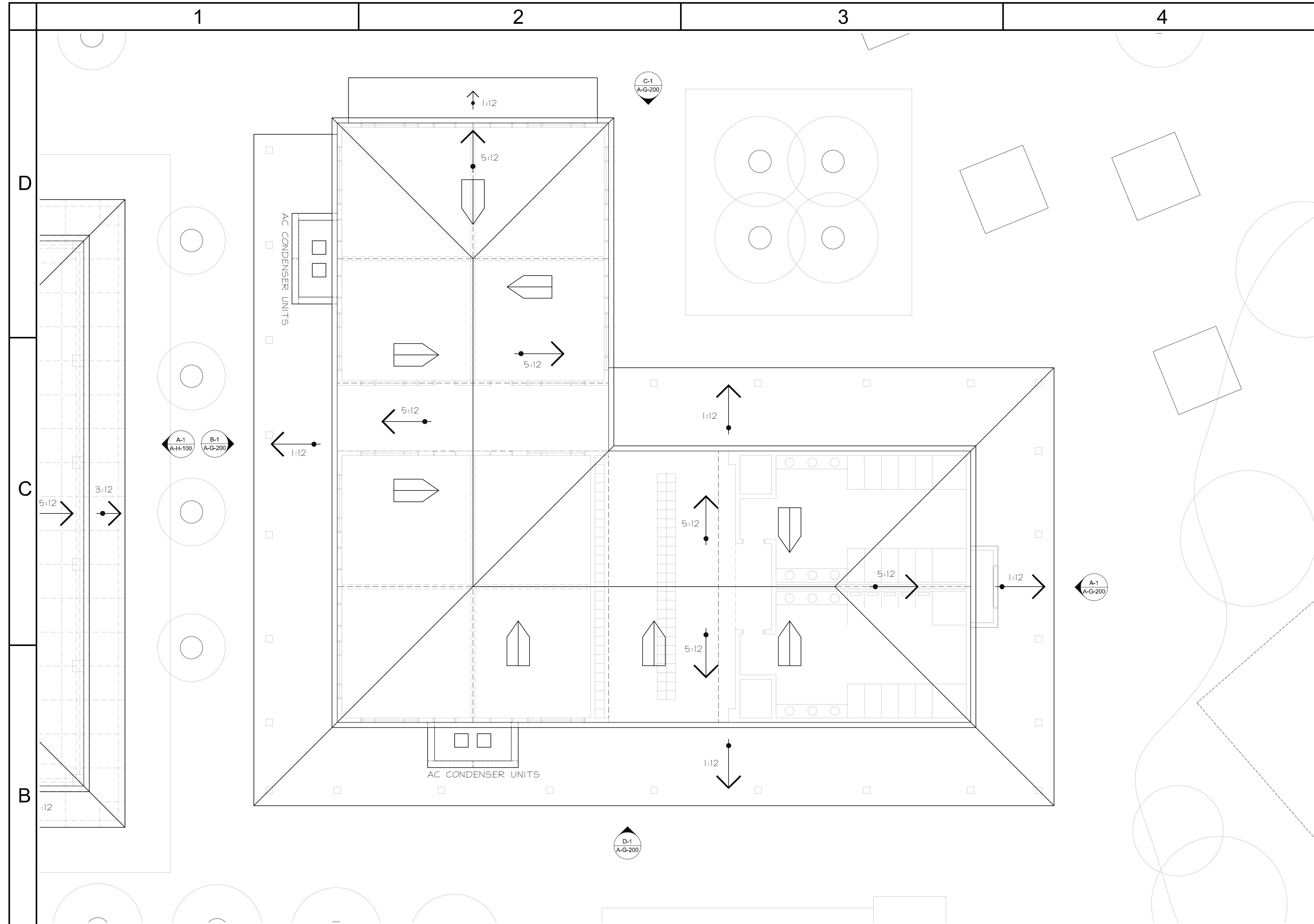
B-1 ROOF PLAN SCALE: 1:100
